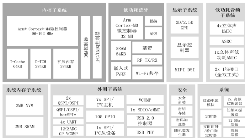
超低功耗Apollo4 Blue Plus SoC的框图
