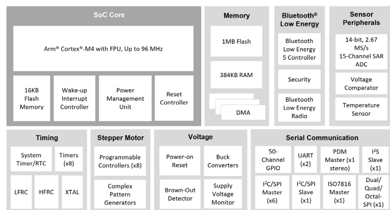
超低功耗Apollo3 Blue SoC的框图
